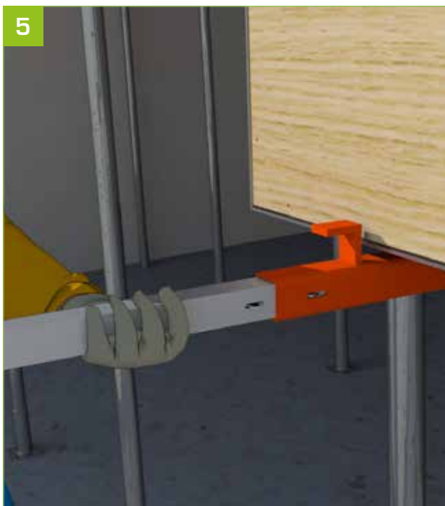
- Enclencher les potelets dans les adaptateurs AlphiSafe pour MaxiDalle.
